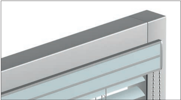
Le store InLine se révèle à la fois fonctionnel et décoratif. Les vis de fixation sont dissimulées derrière le profilé de recouvrement inséré dans le rail.
