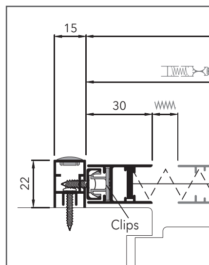
Montage frontal
